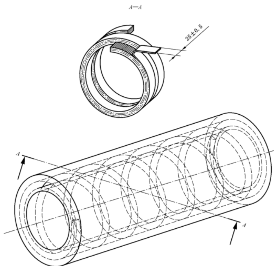
图 7 7 型试样
