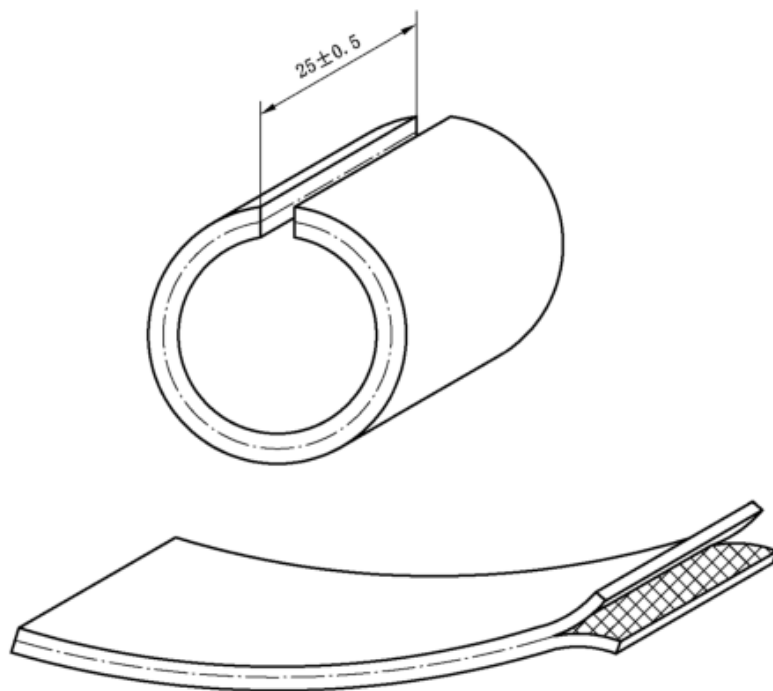
图 1 1 型试样
