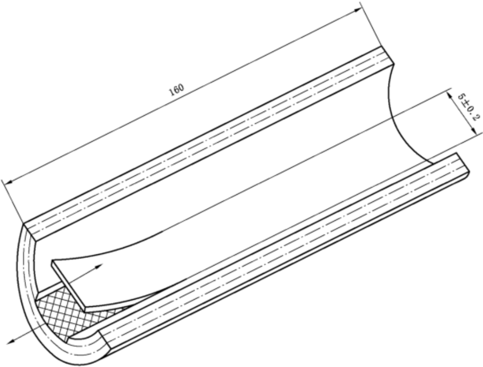
图 5 5 型试样
