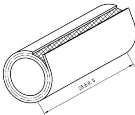
图 8 8 型试样
